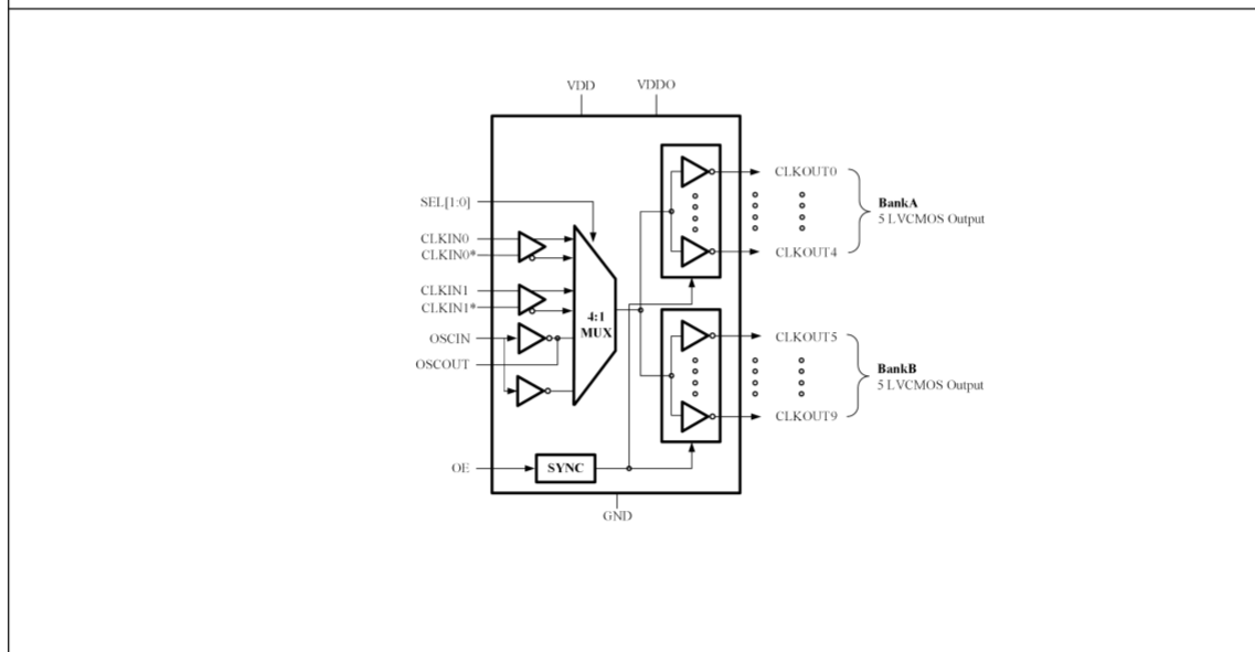
功能示意框图
